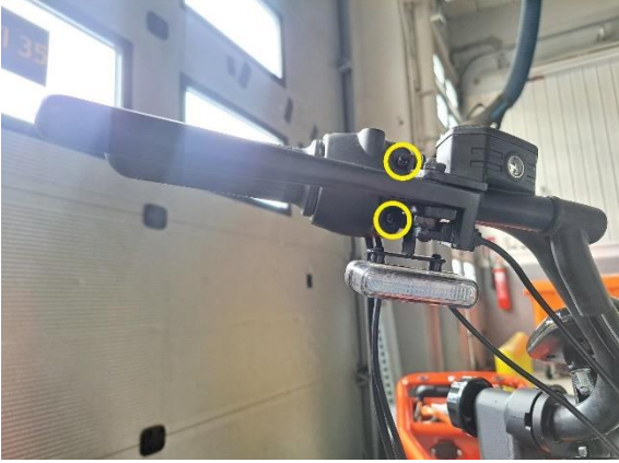
Irrota kaasukahvan kiinnitysruuvit (ristipäämeisseli ph2).
