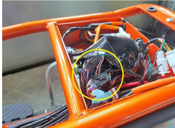
Avaa kaasukahvalle menevät liittimet.
